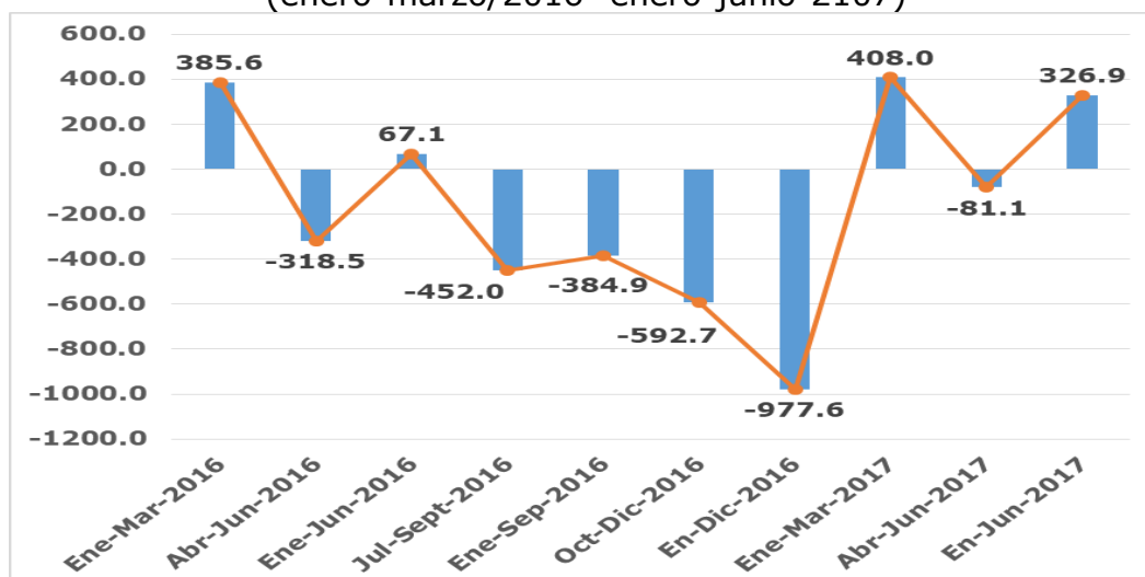
Gráfico 2 Evolución trimestral de la cuenta corriente (Millones de dólares) (enero-marzo/2016- enero-junio-2107)
